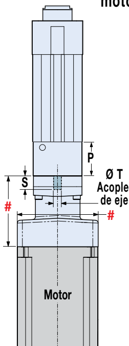
LM Montaje del motor
