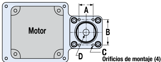
RP Montaje del motor
